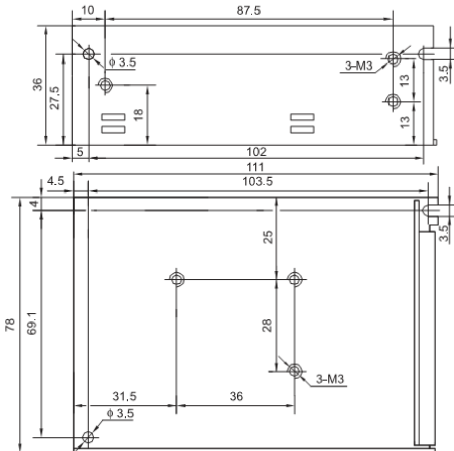
外型结构图:
